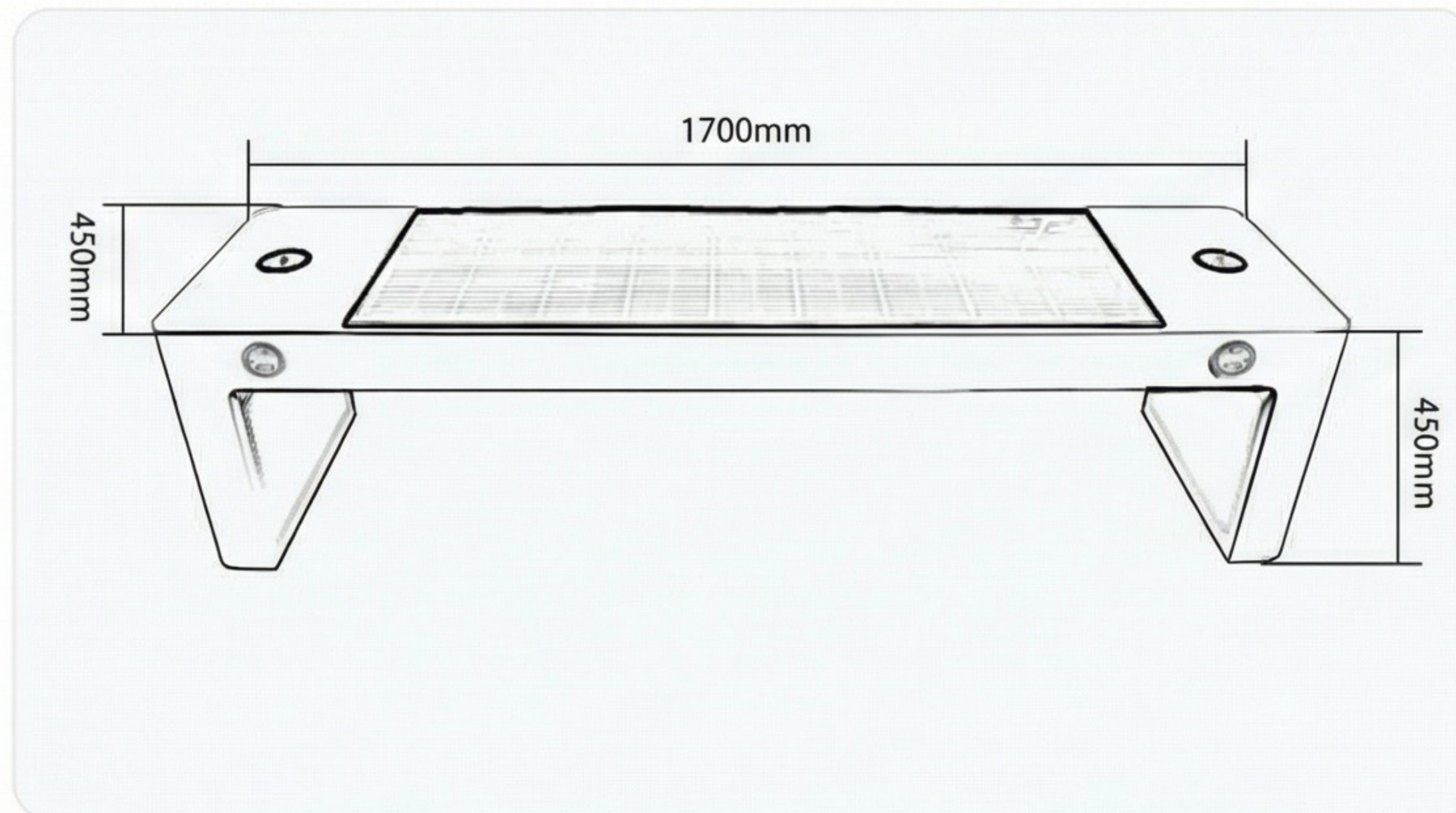
TECHNICKÝ NÁKRES
